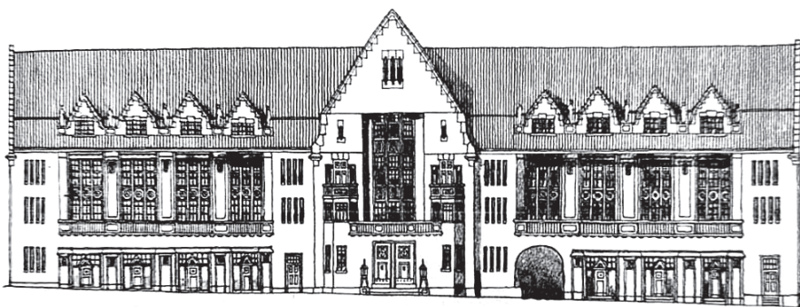
Wachtel Elemér – Rerrich Béla: A kolozsvári városháza és Vigadó terve. A Vigadó főhomlokzata, 1910.
